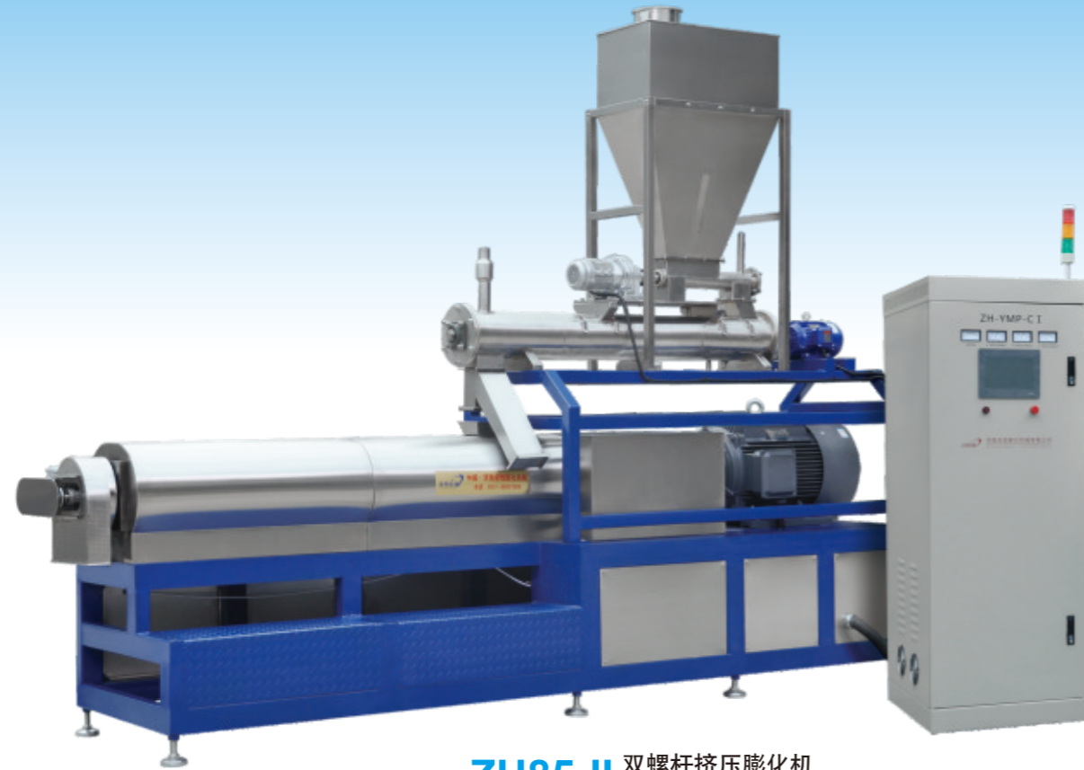
ZH85-II 双螺杆挤压膨化机 Double-screw Extruder
